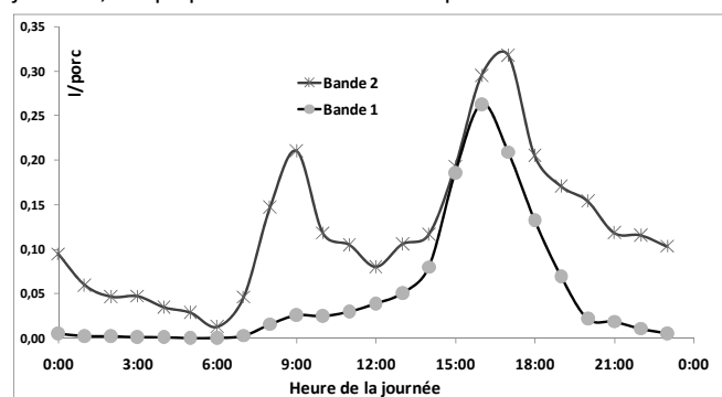
Figure 1 - Evolution journalière de la consommation d'eau
