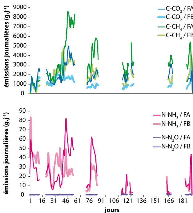
Figure 2 : Variations des émissions journalières carbonées et azotées mesurées de la fosse
